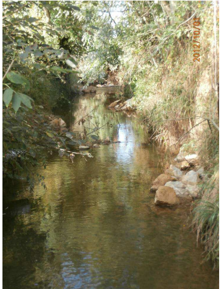
Réalisation 2012 : apport de graviers et de blocs en alternant rive droite/ gauche/ milieu du lit afin de diversifier le milieu
