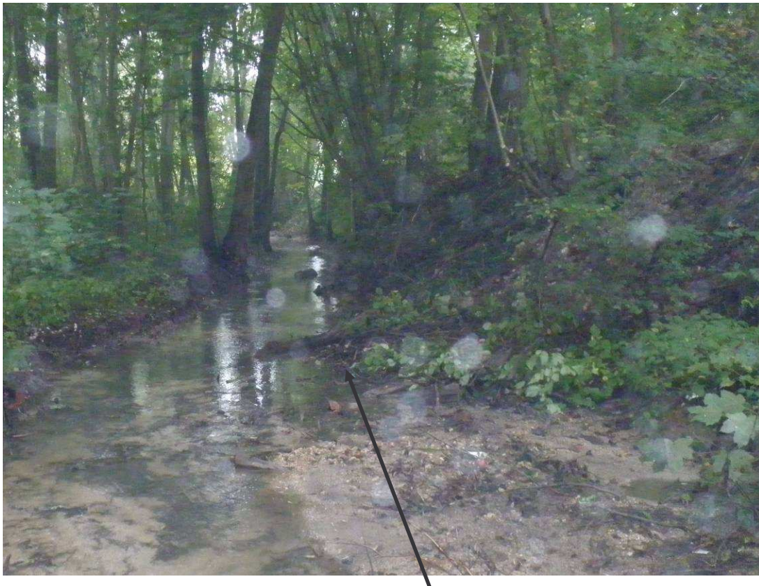
Embâcle traitée et confection d'un peigne en rive gauche accentuant le léger méandre
